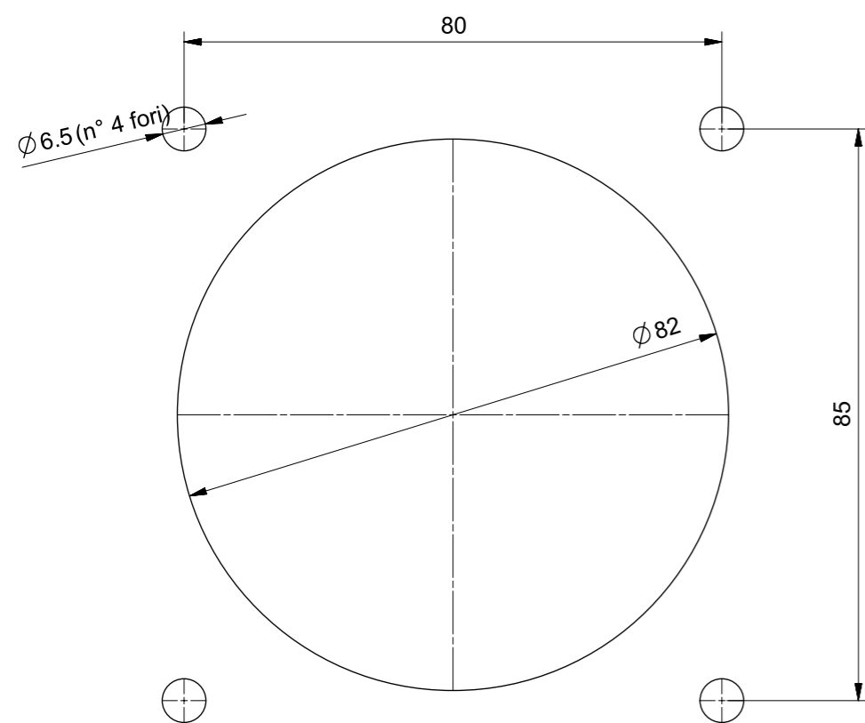
Dima di foratura
