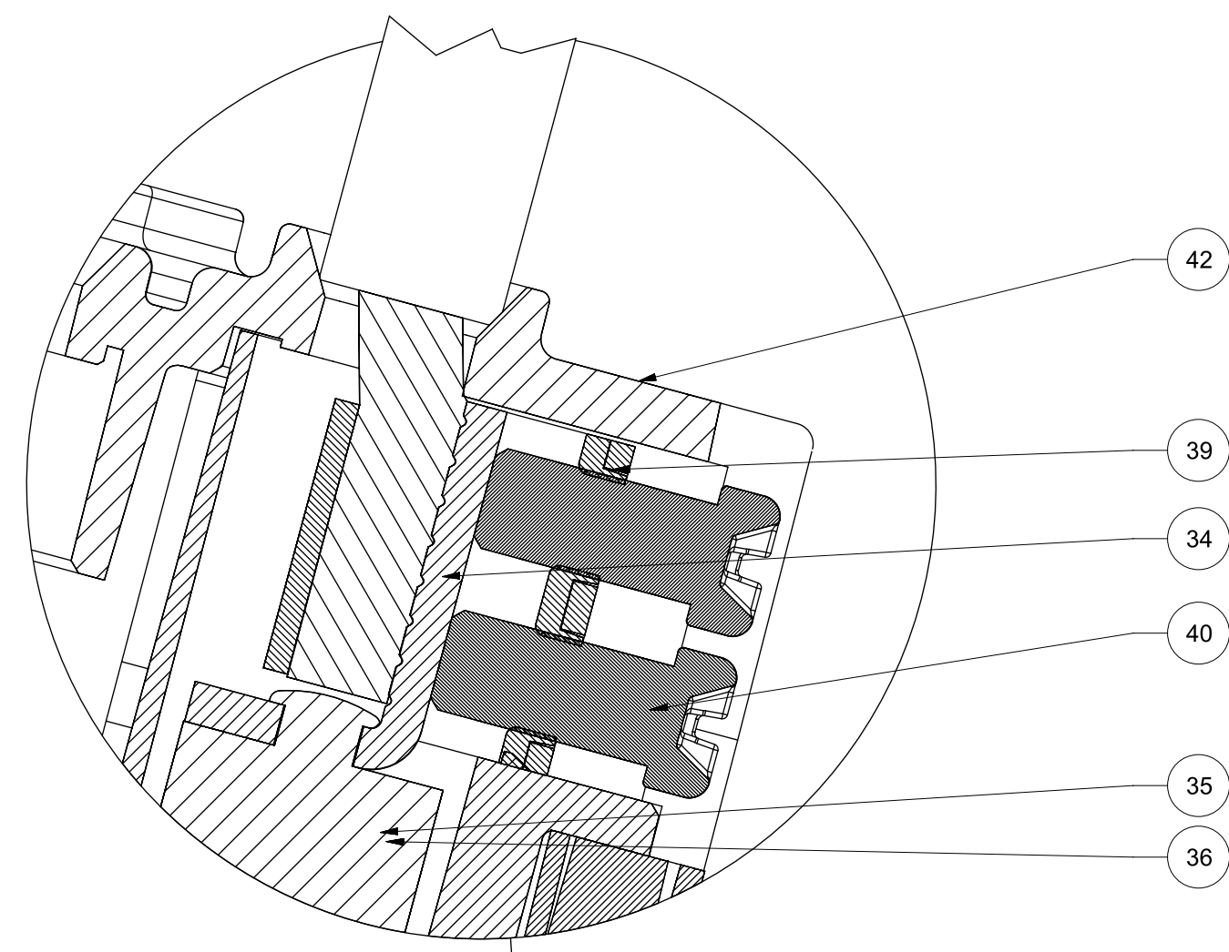
PARTICOLARE SERRAGGIO CAVO SCALA 3:1
