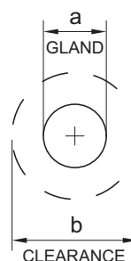
Fig. 2 IT: Distanza Minima e dimensione pressacavo. EN: Cable gland dimension and minimum distance. FR: Distance minimum et dimension presse-étoupe ES: Distancia mínima y dimensión prensacable
