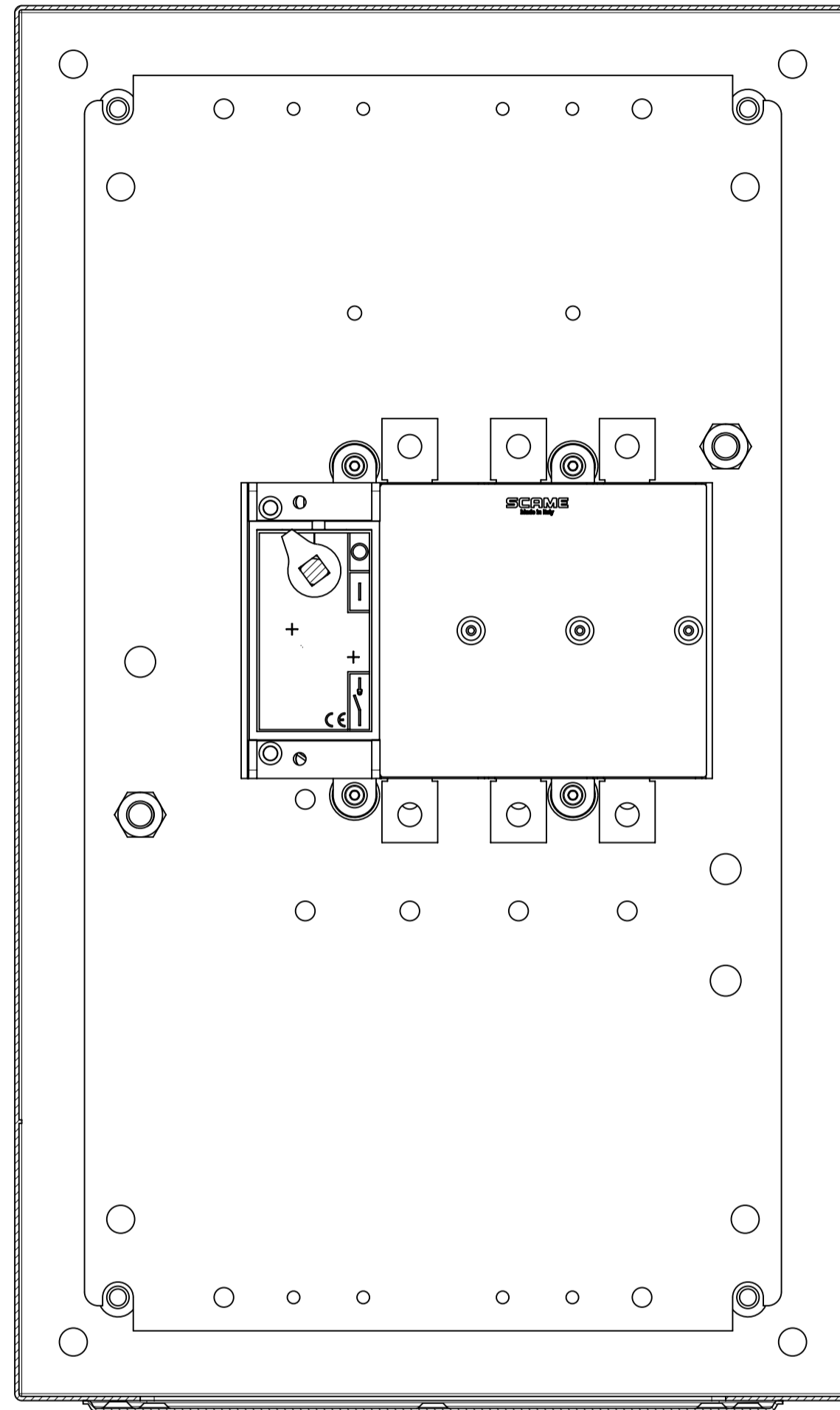
Sezione A-A
