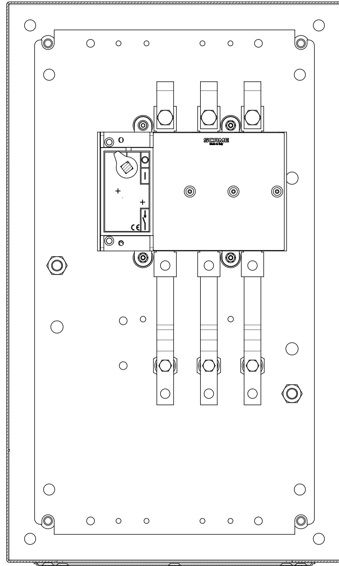
Sezione A-A
