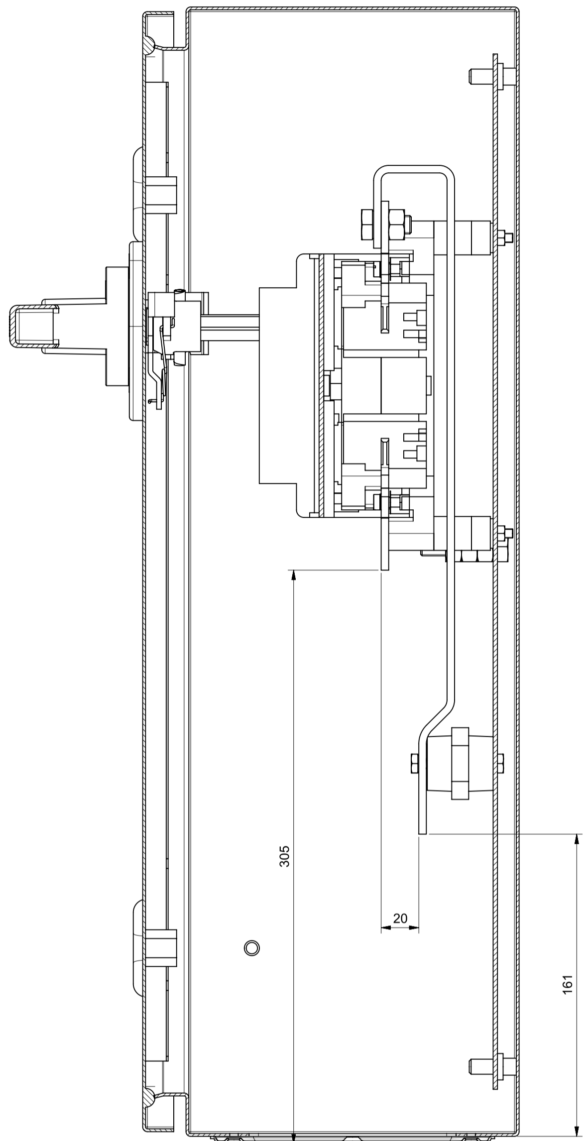
Sezione B-B
