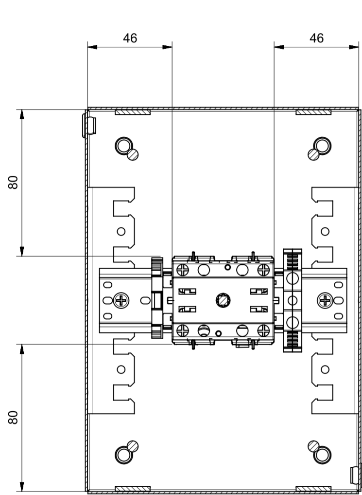
Sezione A-A
