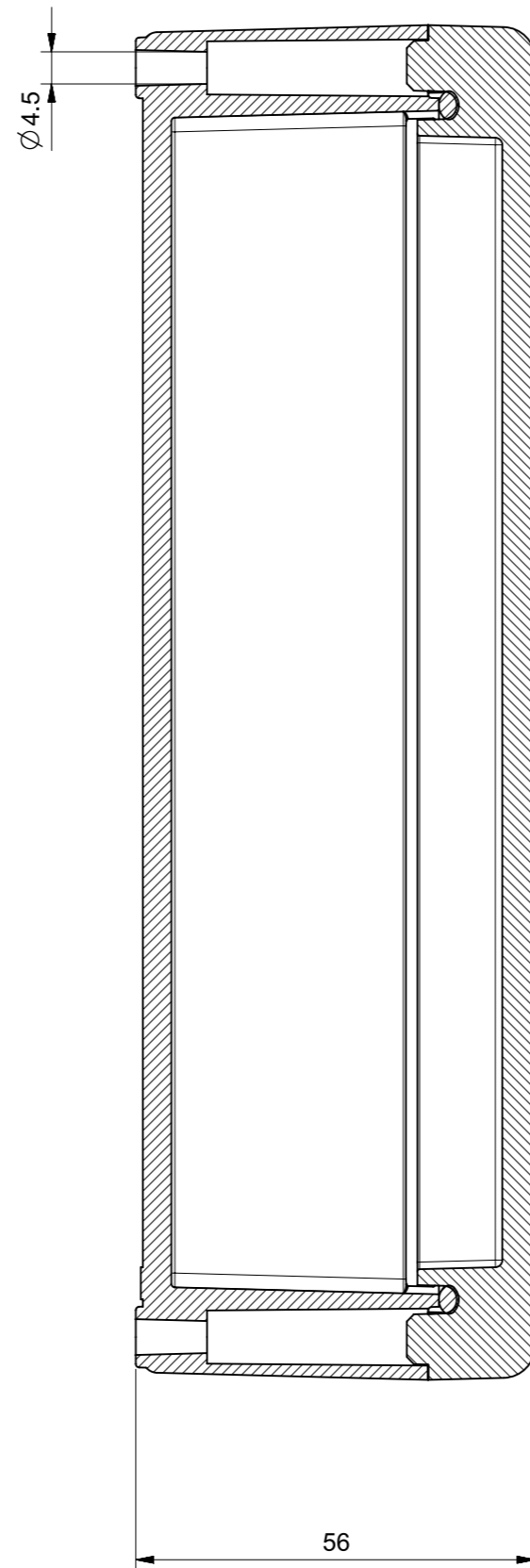
Sezione B-B
