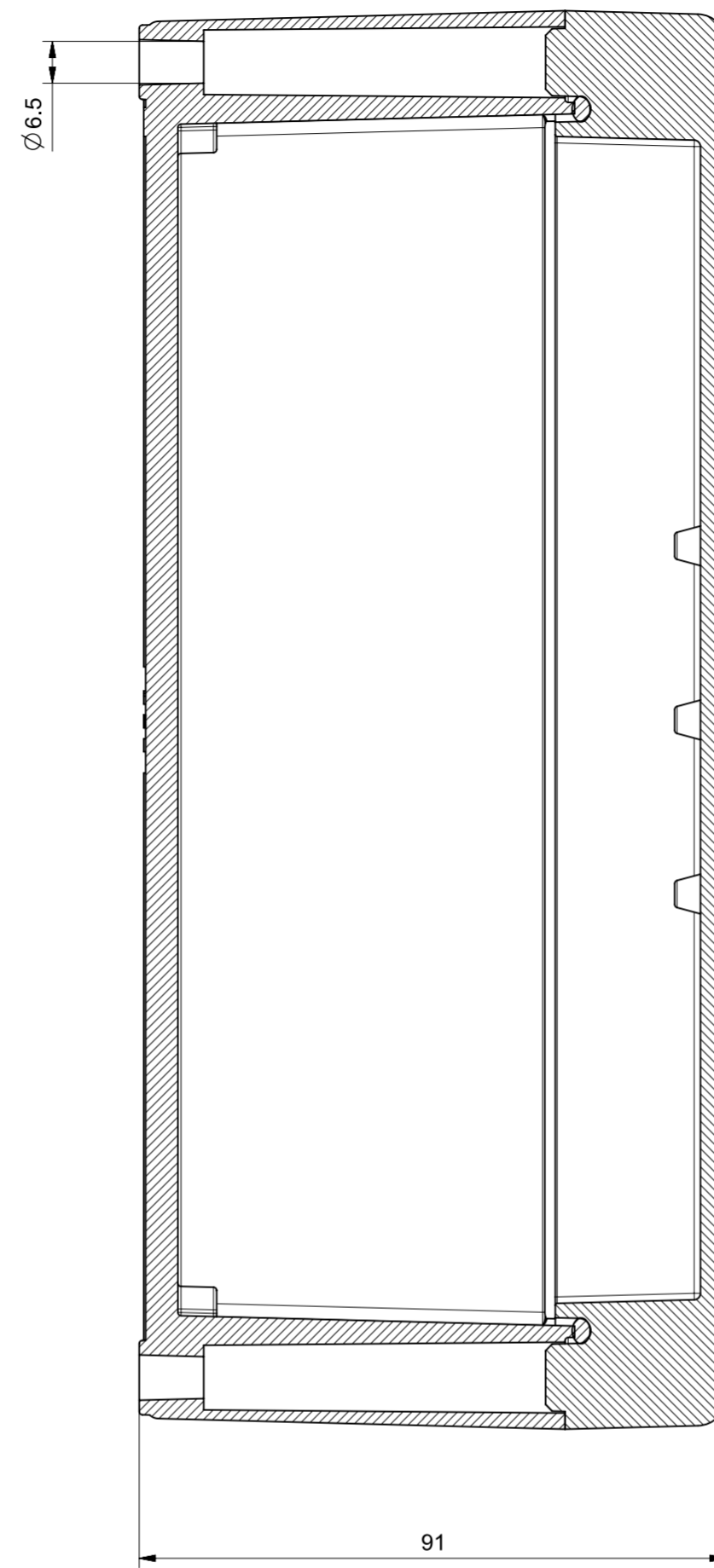
Sezione D-D
