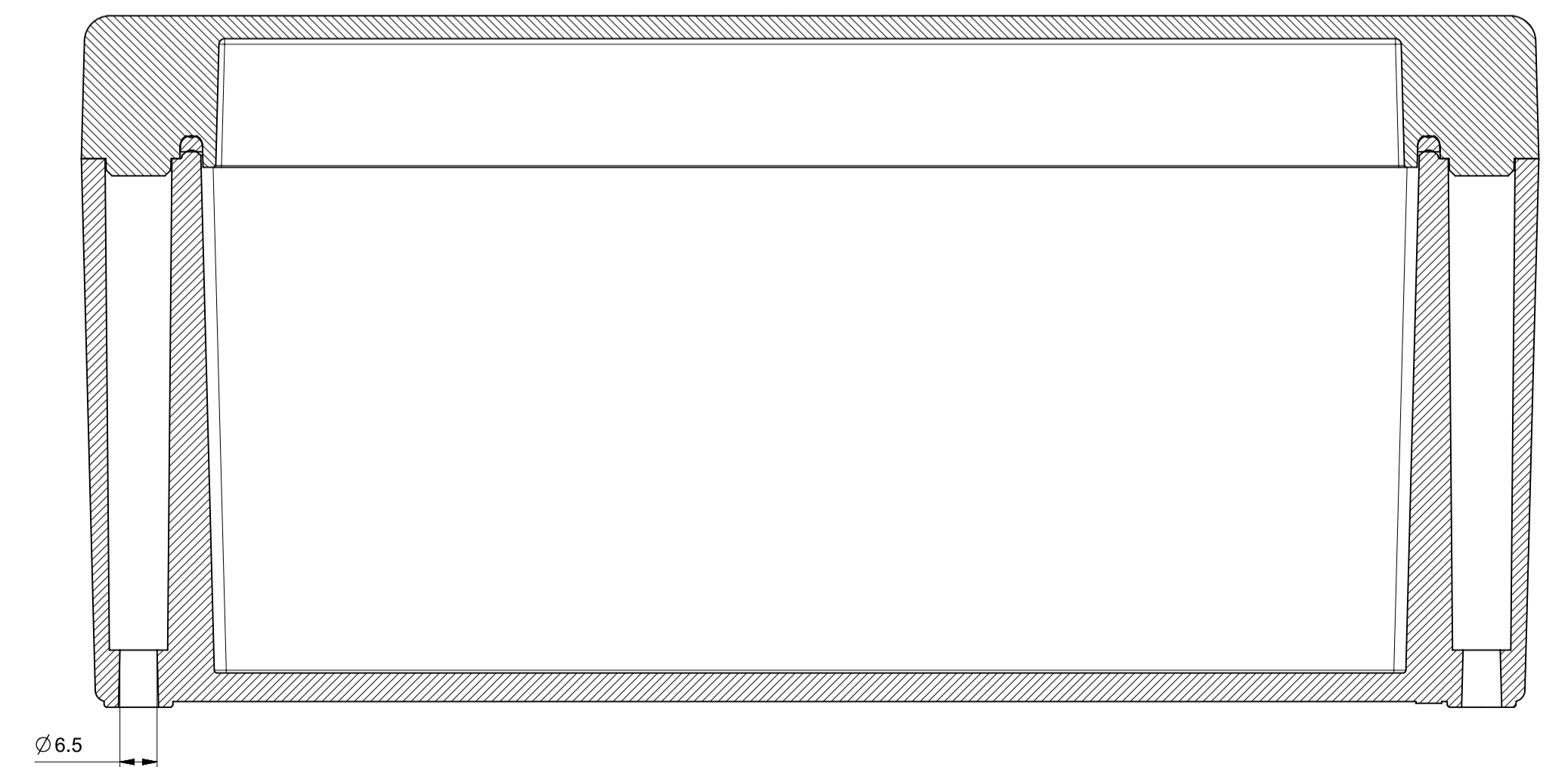
Sezione B-B
