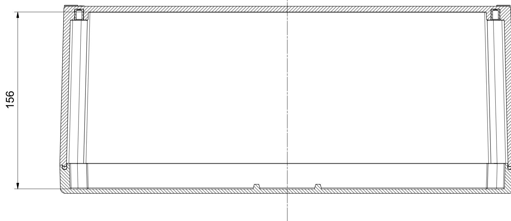
Sezione A-A
