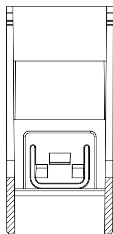
Sezione B-B
