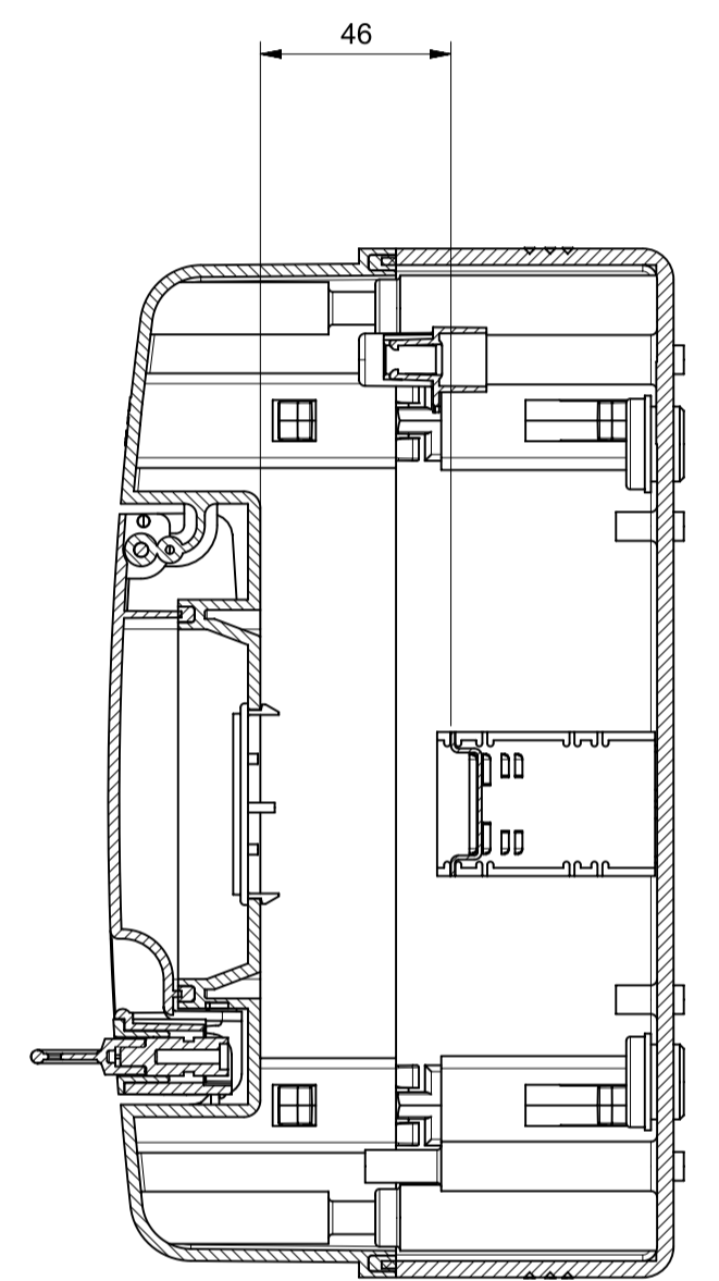
Sezione A-A
