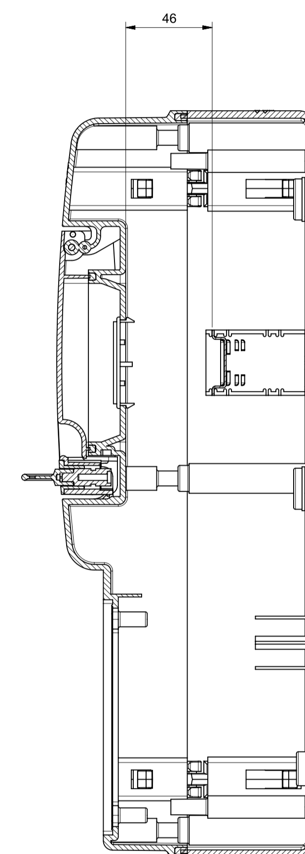
Sezione A-A
