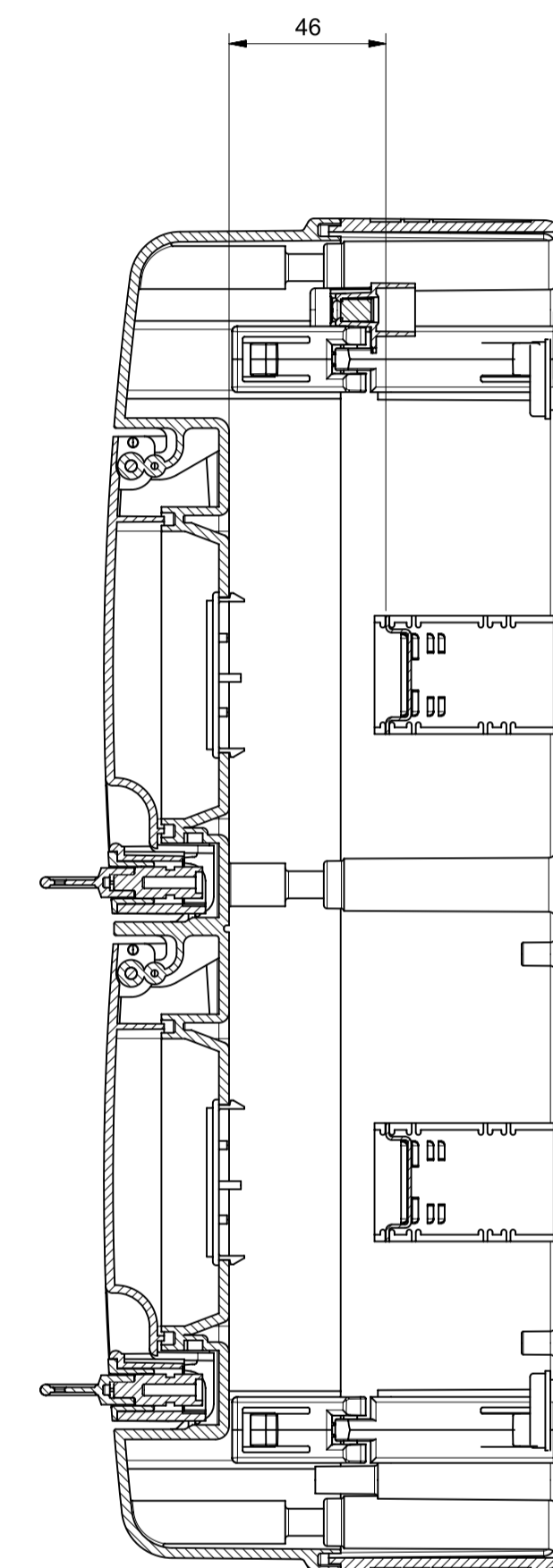
Sezione A-A
