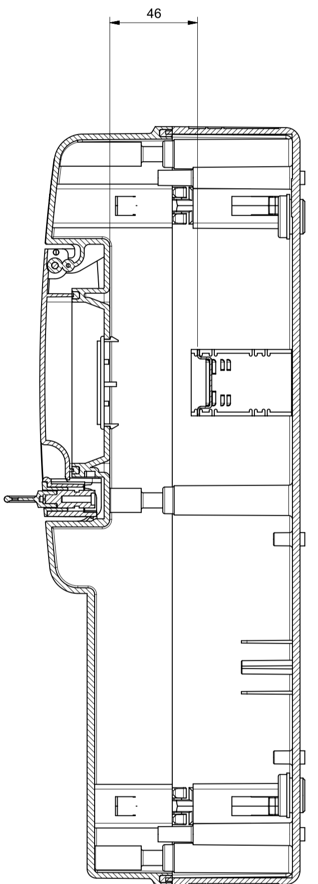
Sezione A-A
