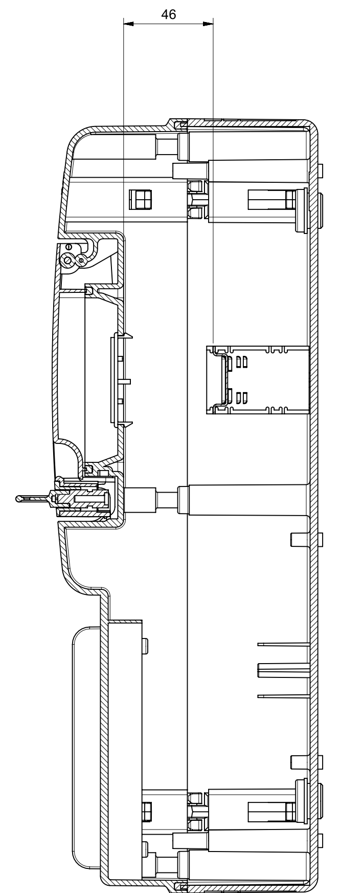
Sezione A-A
