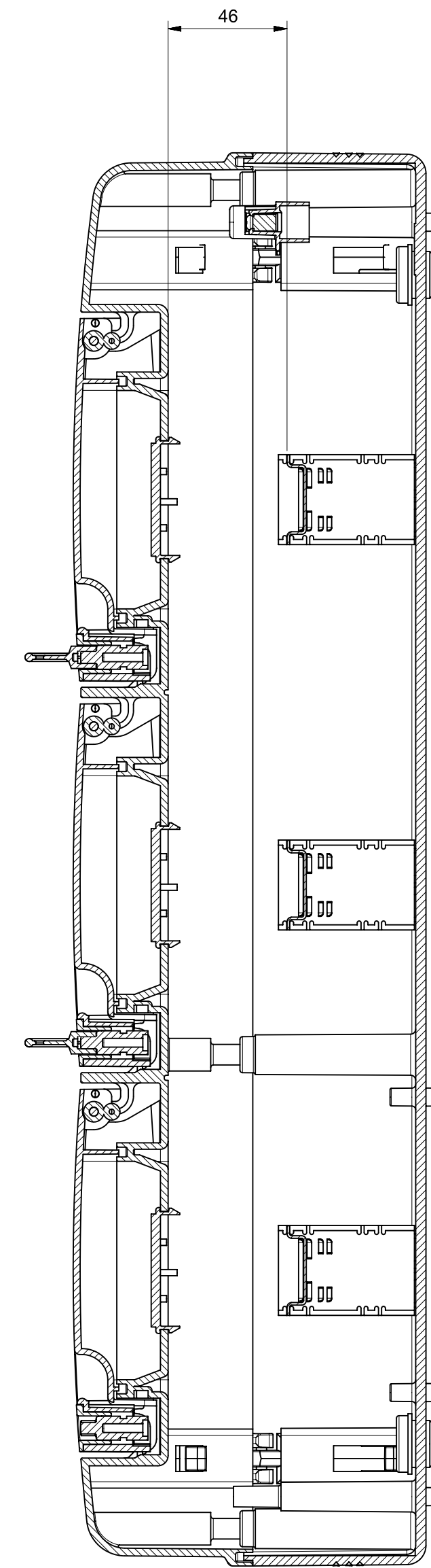
Sezione A-A
