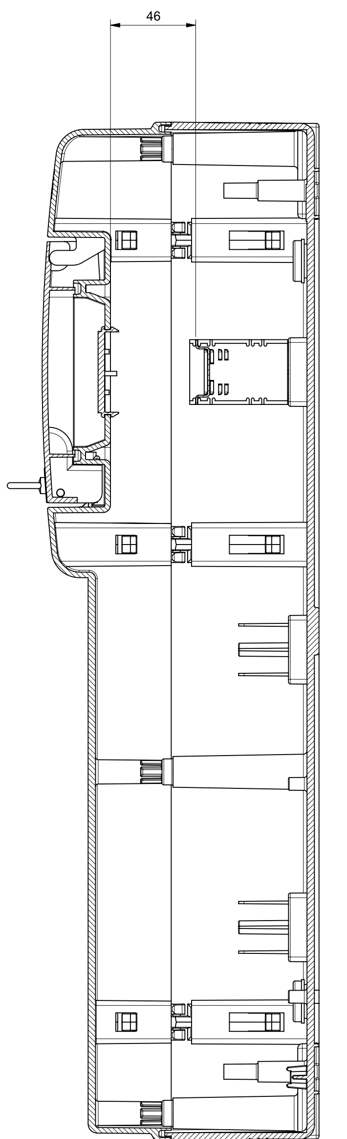
Sezione A-A
