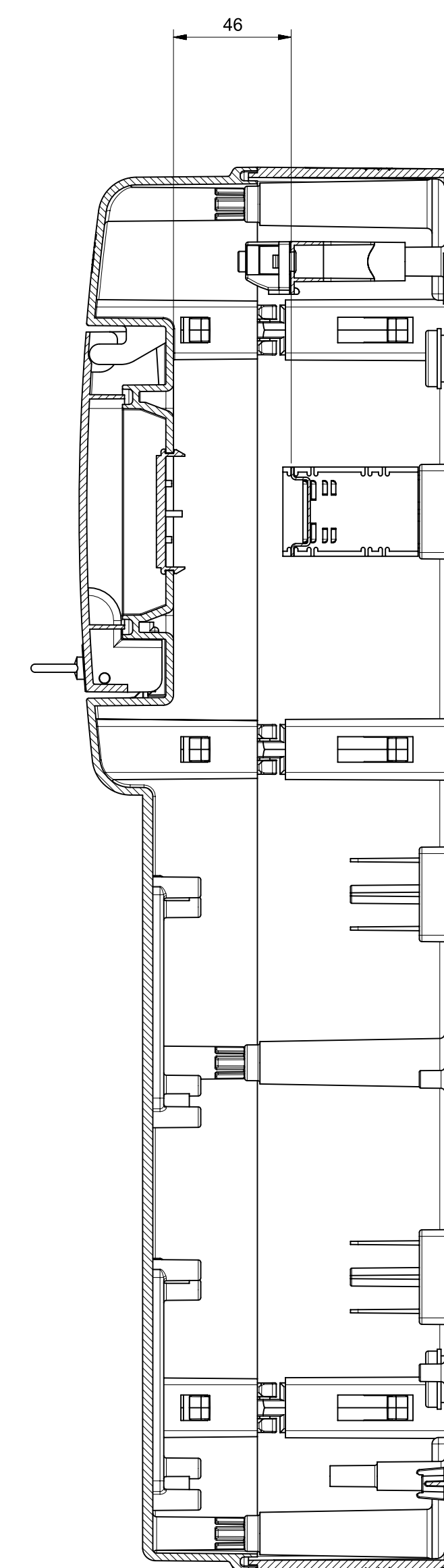
Sezione A-A
