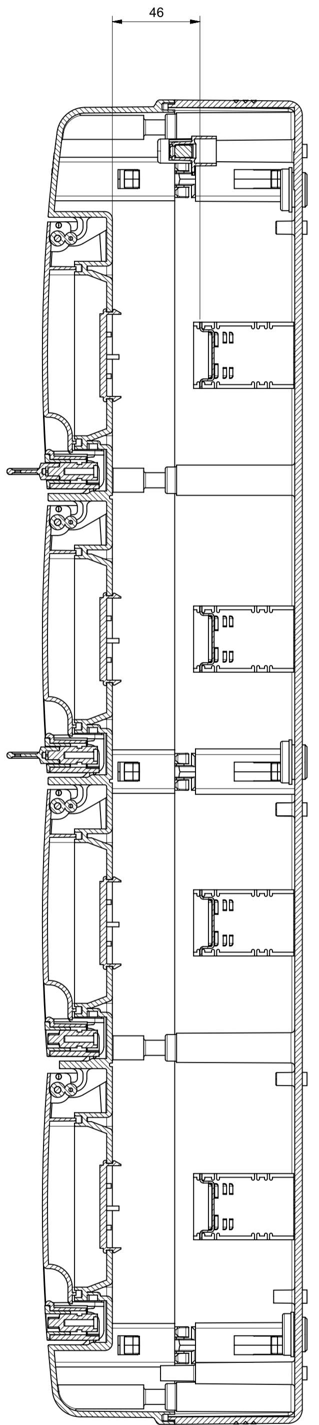
Sezione A-A
