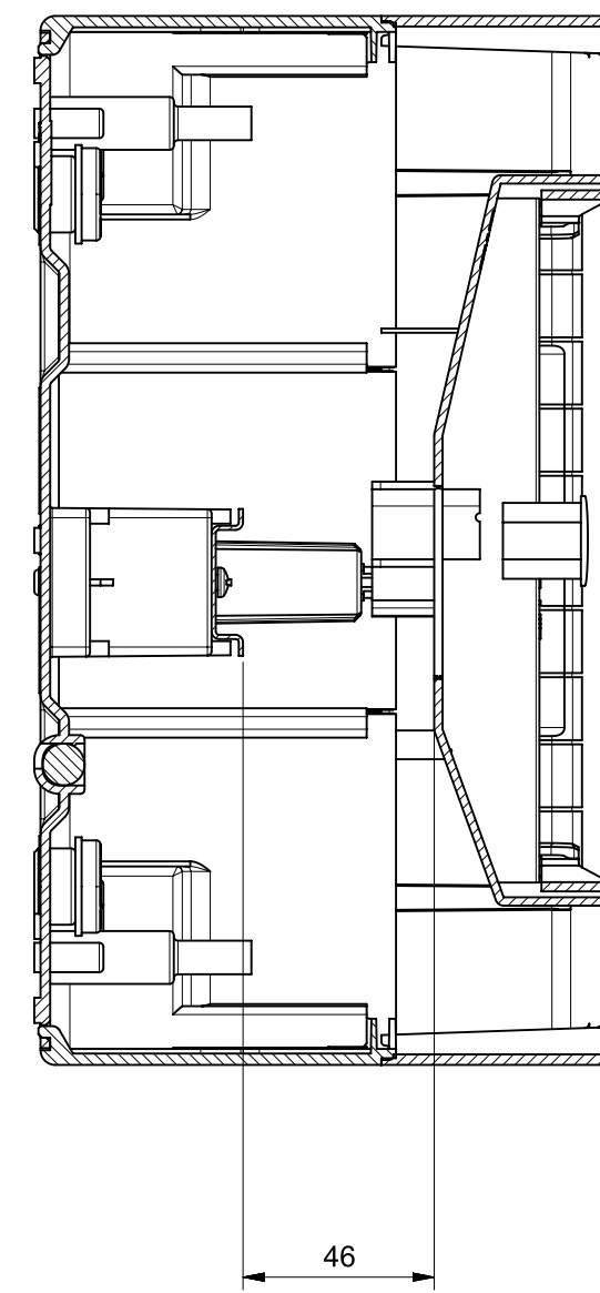
Sezione A-A
