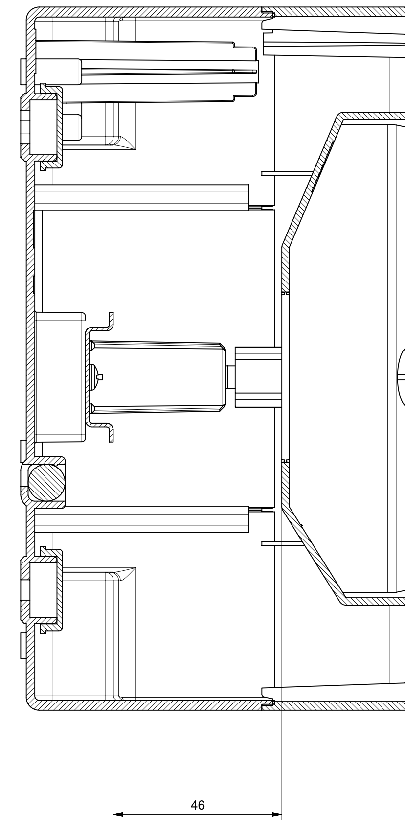
Sezione A-A
