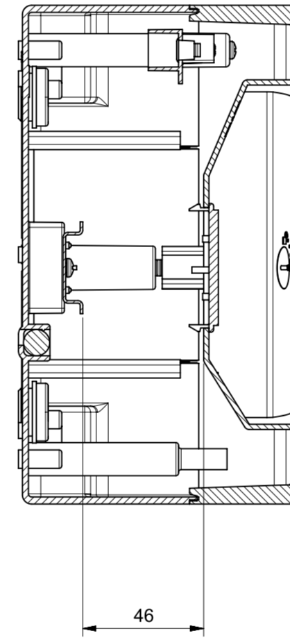
Sezione A-A
