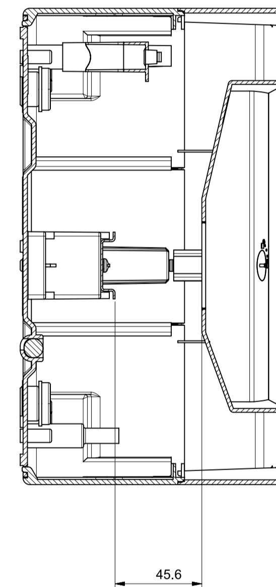
Sezione A-A
