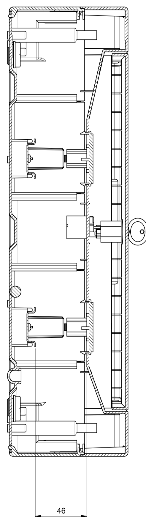
Sezione A-A
