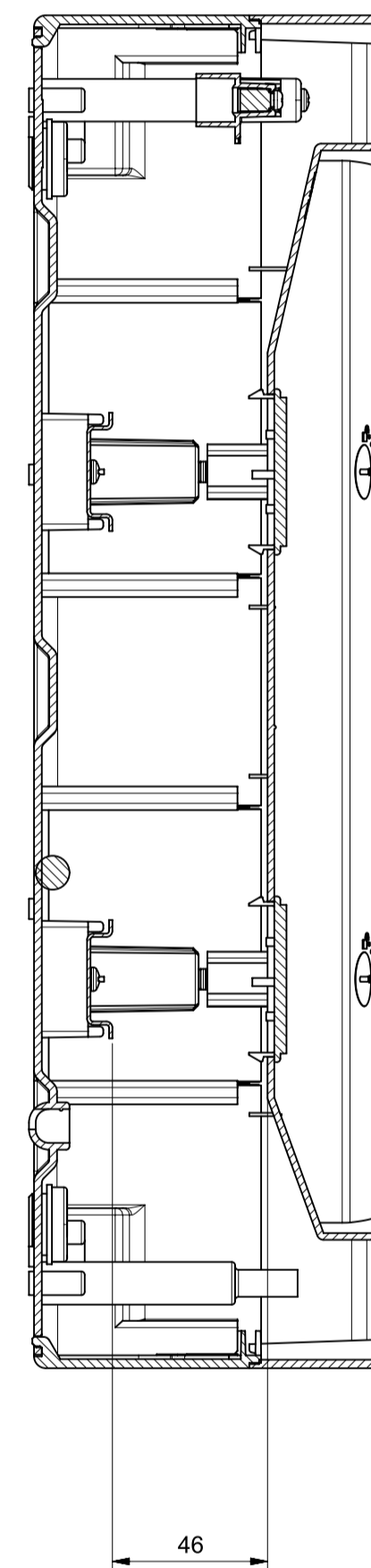
Sezione A-A
