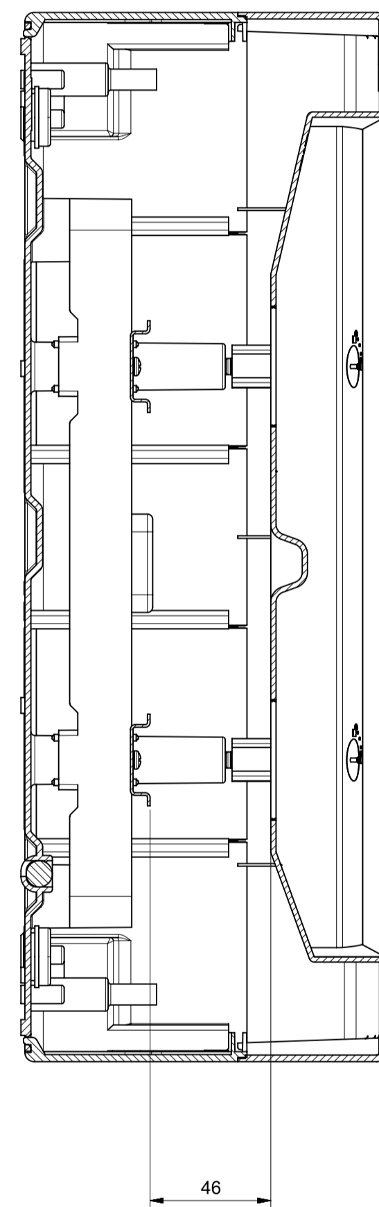
Sezione A-A
