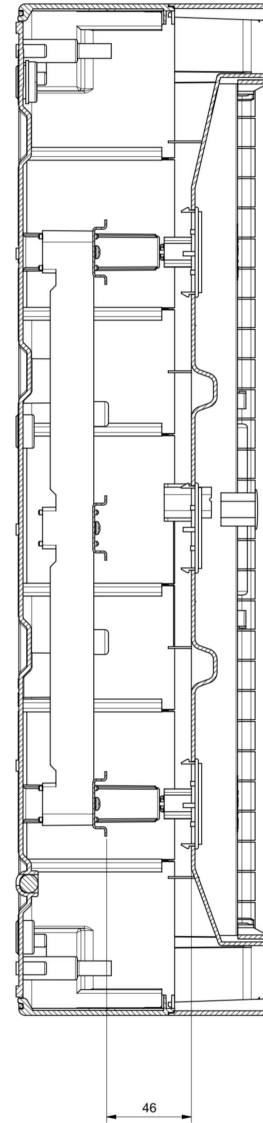
Sezione A-A
