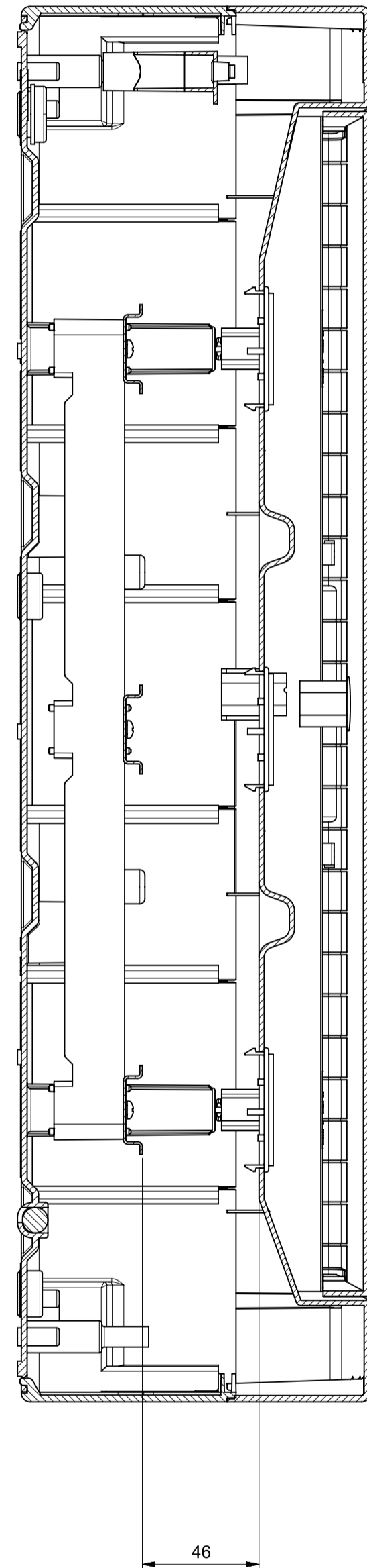
Sezione A-A
