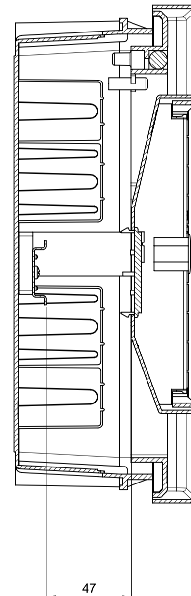
Sezione A-A
