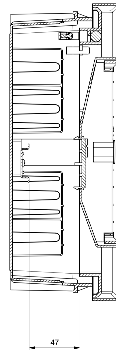
Sezione A-A
