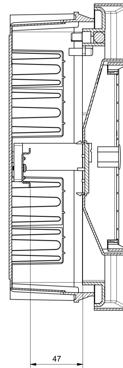
Sezione A-A
