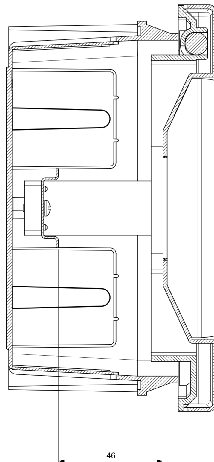
Sezione A-A
