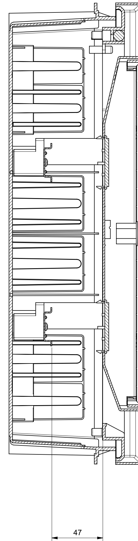
Sezione A-A
