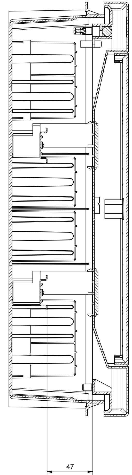
Sezione A-A
