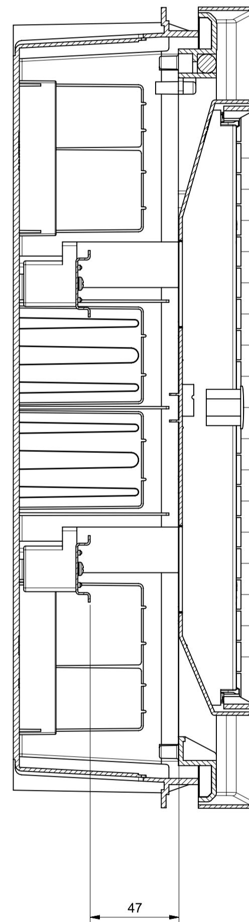
Sezione A-A
