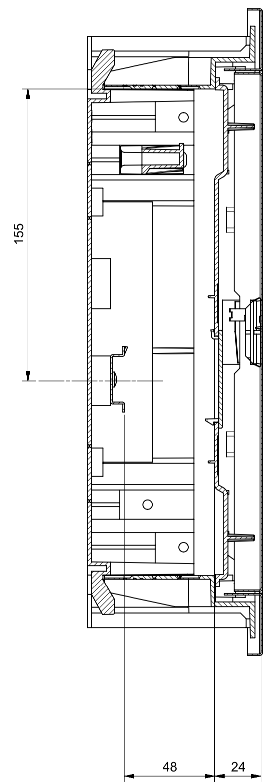
Sezione A-A
