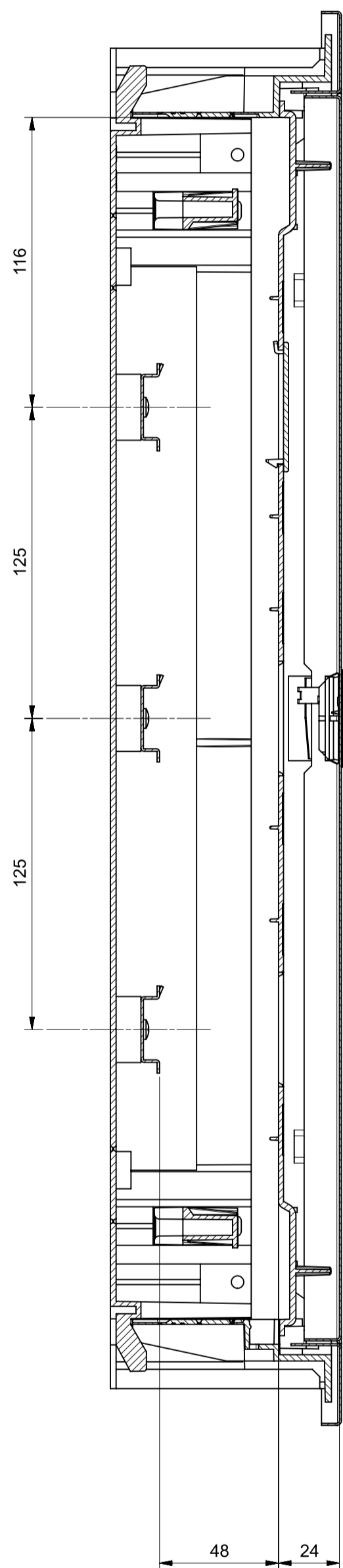
Sezione A-A
