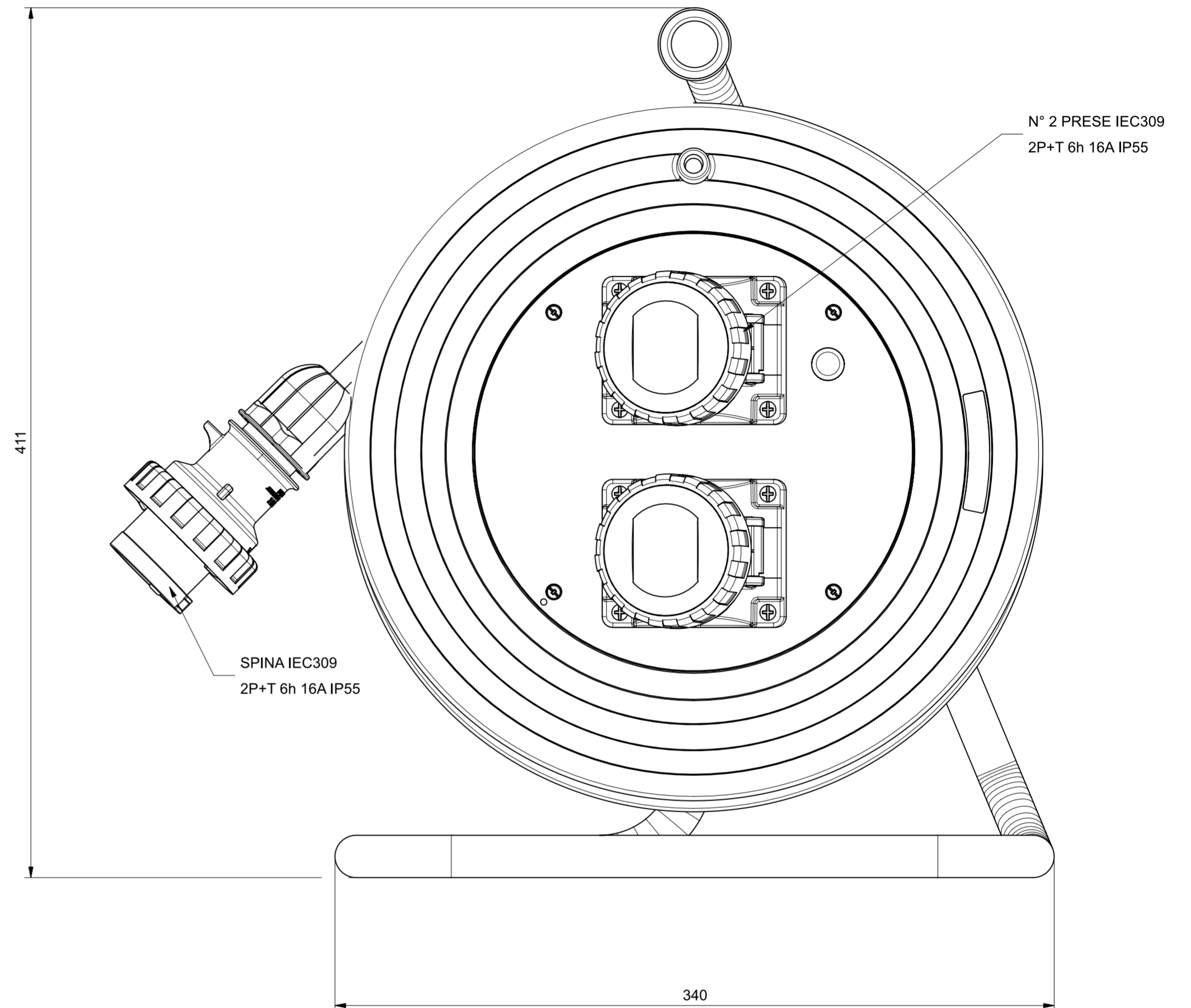
L'AVVOLGICAVO 746.3510-1593 HA SPINA E PRESE CON RIFERIMENTO ORARIO 4h
