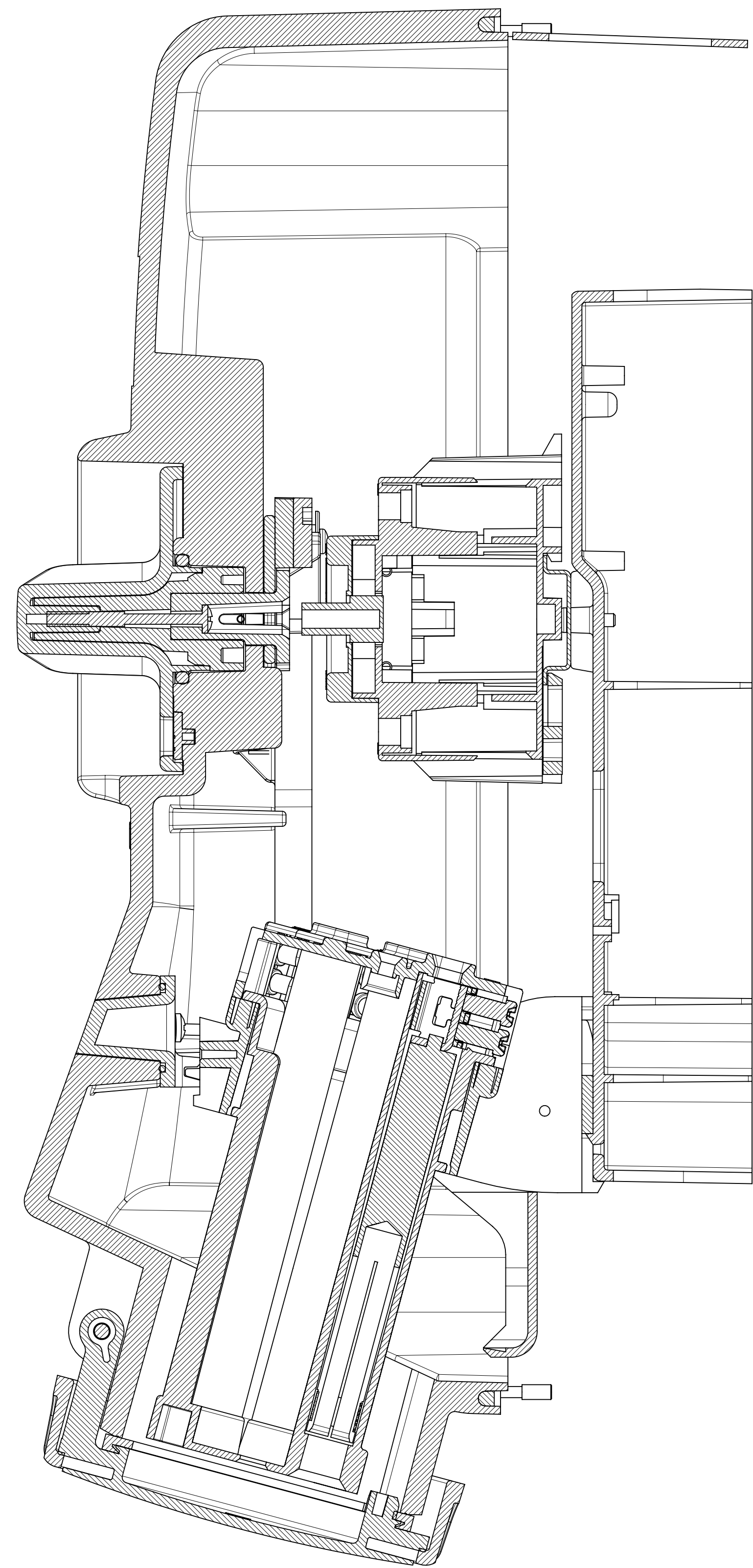
Sezione A-A
